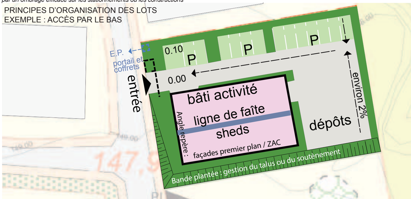
Principe d'implantation - Accès au lot par le bas - UEa1
